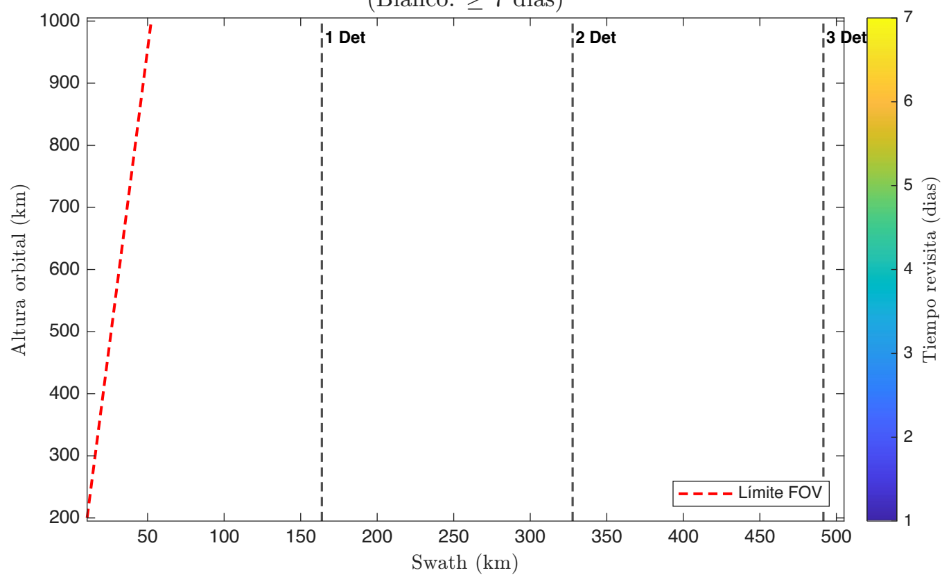
Tiempo Revisita - 1 Satelite(s); 1 Telescopio(s): Korsch; Detector 2 (Blanco: \geq 7 dias)
